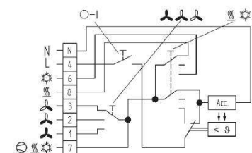
KLR-E 7038 kapcsolási rajza:
